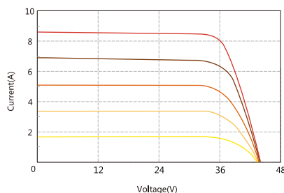
UL300M-72 出力特性図
